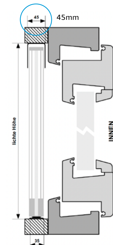
Vertikalschnitt
