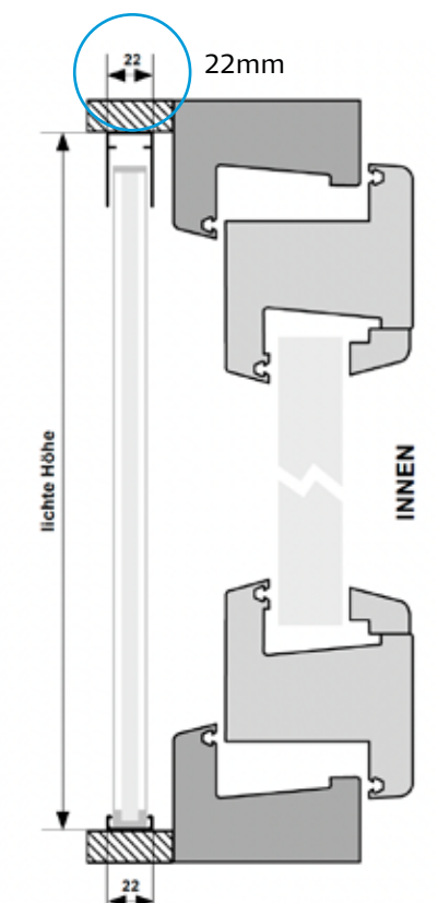
Vertikalschnitt
